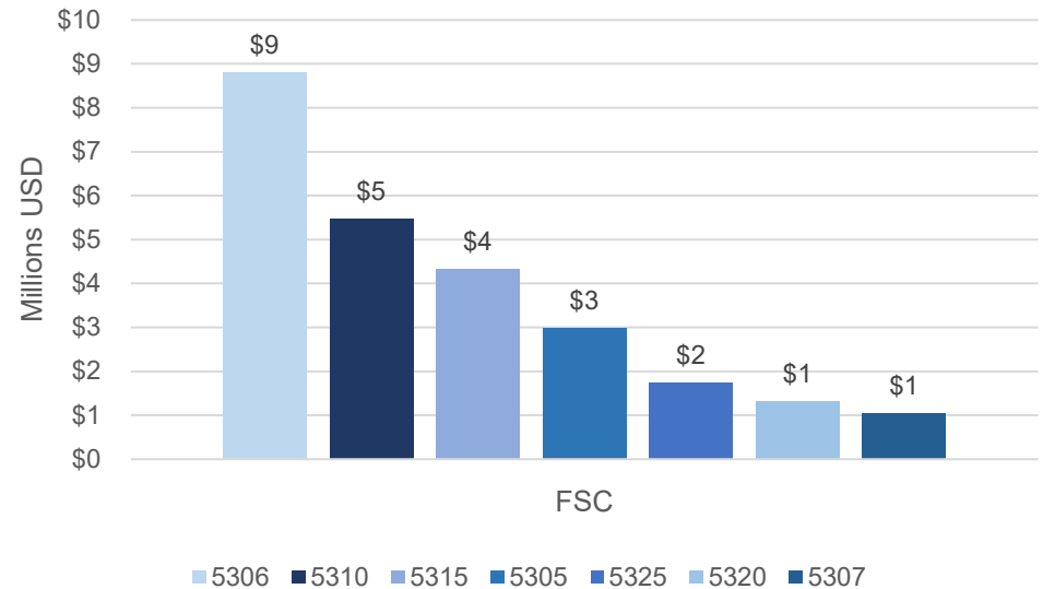
Backorder Valuation
